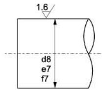
相配轴 Mating Shaft
